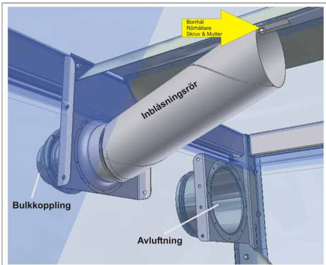
Figur 28: Inblåsningröret
