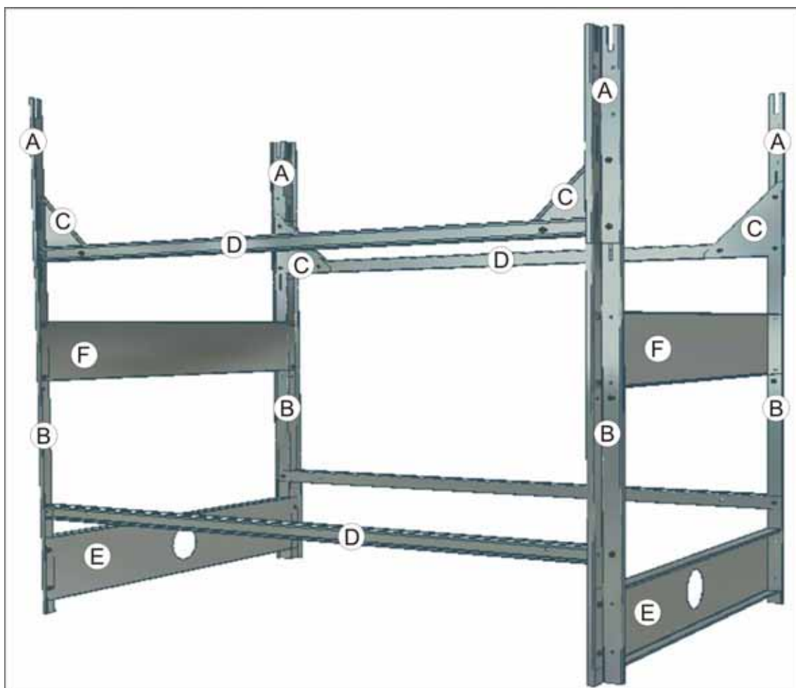
Figur 7: Förrådsstativ
