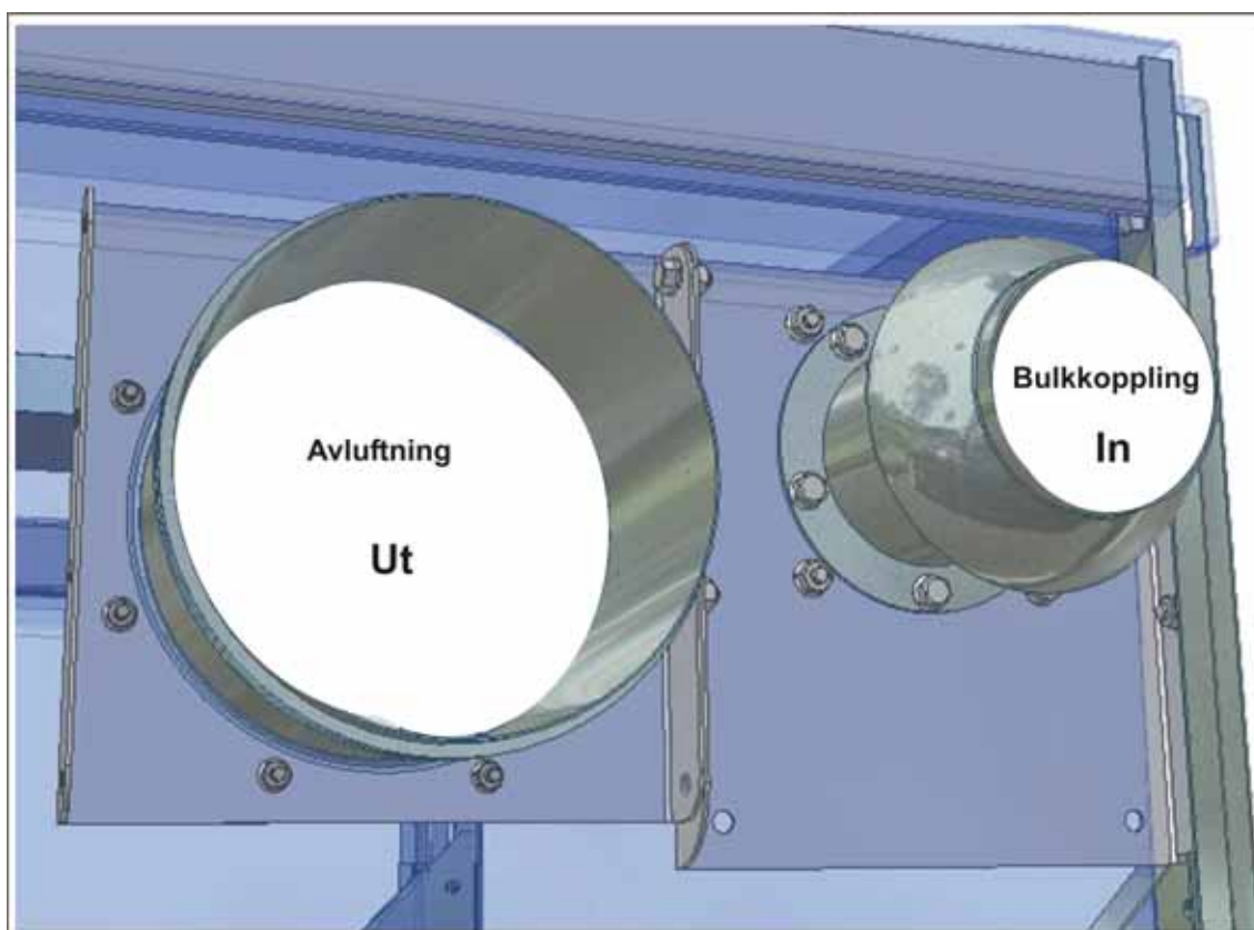
Figur 29: In- utblås
