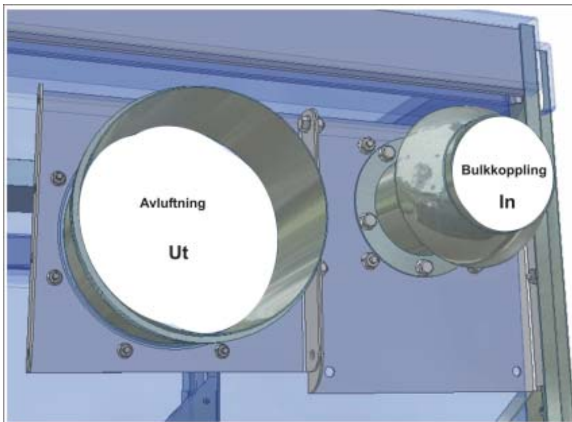
Figur 5: In- utblås
