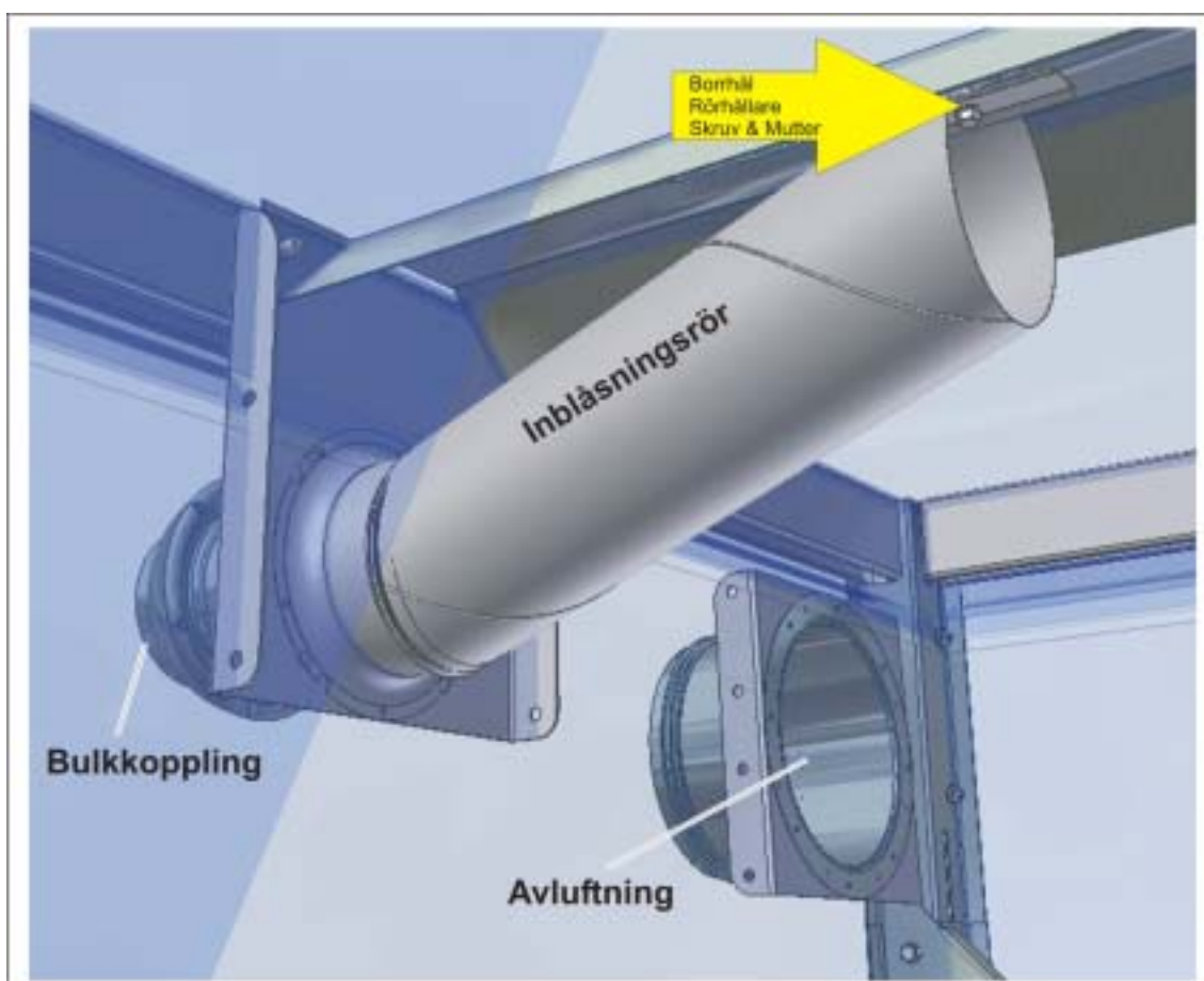
Figur 4: Inblåsningsröret
