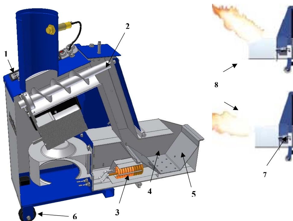
Figur 3 Pelletsbrännaren Flex-a
