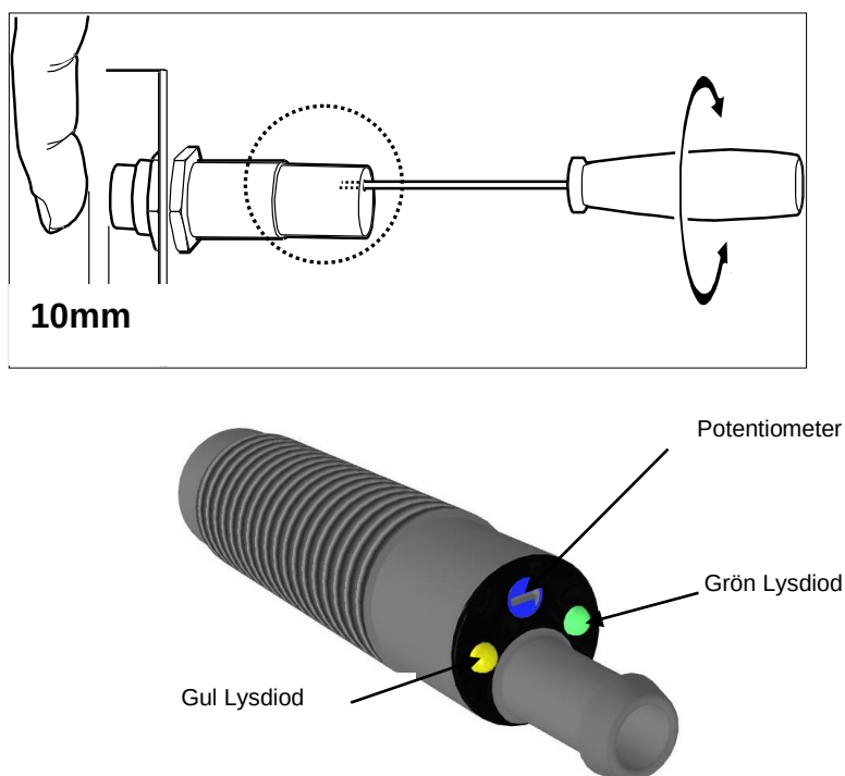
Figur 6 Nivågivare
