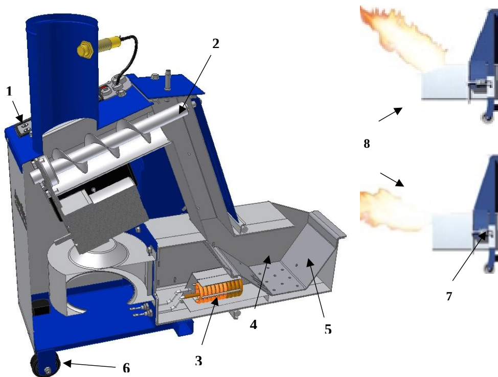
Figur 3 Pelletsbrännaren Flex-a
