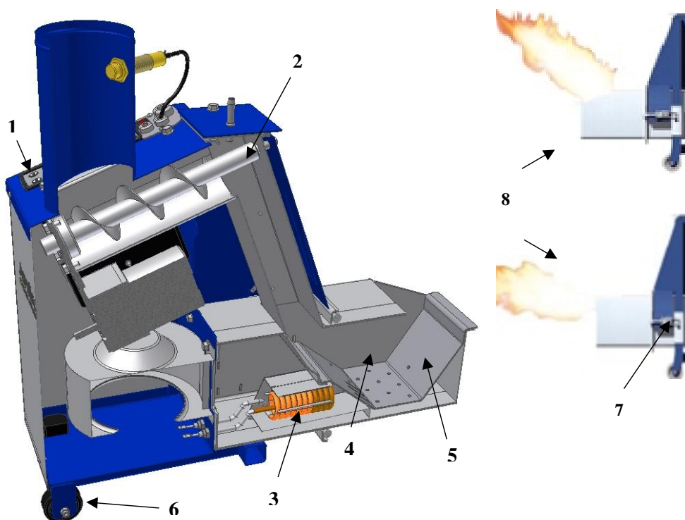
Figur 3 Pelletsbrännaren Flex-a
