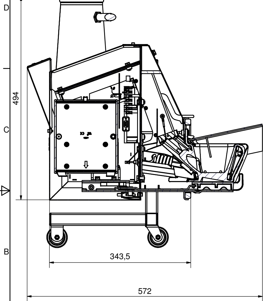
A-A (0,25 : 1)
